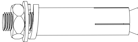
U M8x70 (x4)
